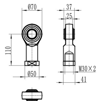
球形铰接KA
