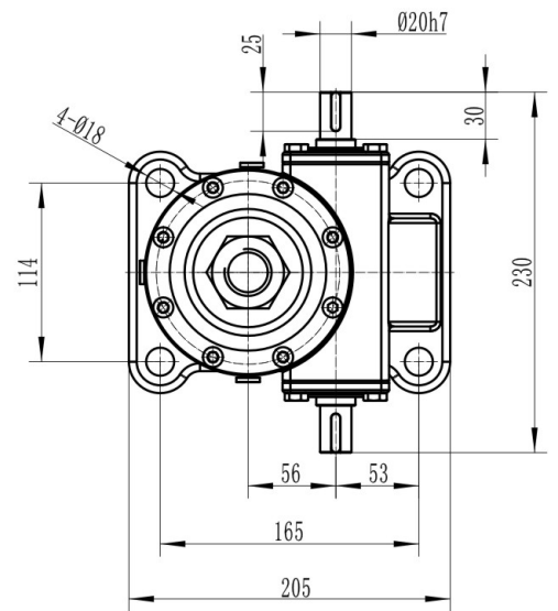
球形铰接KA
