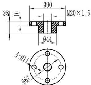
法兰端BP
